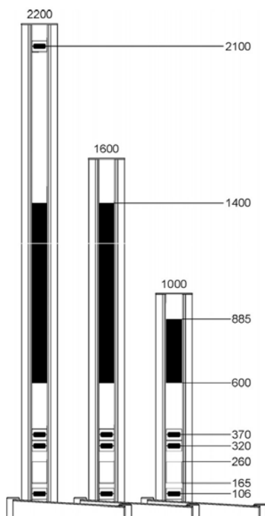
↑ Расположение кабельных разъемов
