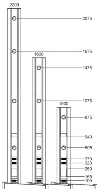
↑ Расположение дополнительных розеток
